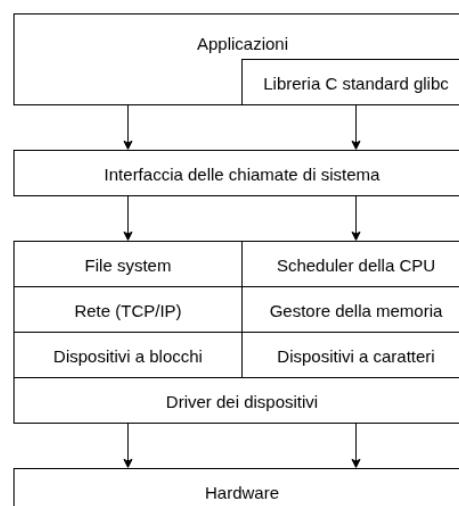
(b) Struttura di Linux
